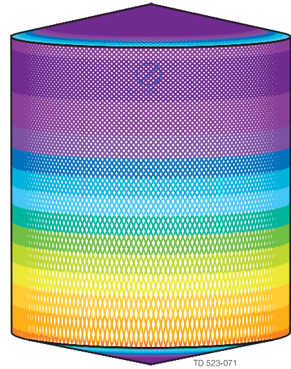
D4,6m H5,5m, Toftejorg TJ 20G, 4 x ø5,5 mm Durée = 8,3 mn, consommation d'eau = 1612 l (428 gallon)
