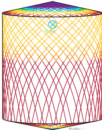
D4,6m H5,5m, Toftejorg TJ 20G, 4 x ø5,5 mm Durée = 2,08 mn, consommation d'eau = 403 l (106 gallon)
