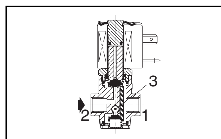
fonction NF (corps laiton)
