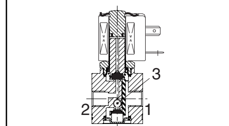
fonction U (corps acier inox)
