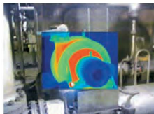
Incrustation d'image
