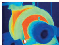
IR integral
