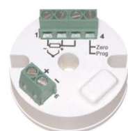
Transmetteur programmable 900 PRO
